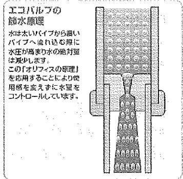
エコバルブの節水原理
